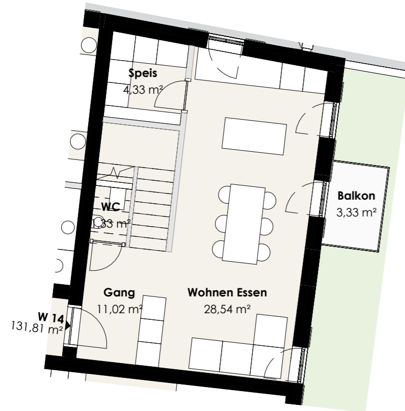
Wohnung 14 - 1. Obergeschoss
